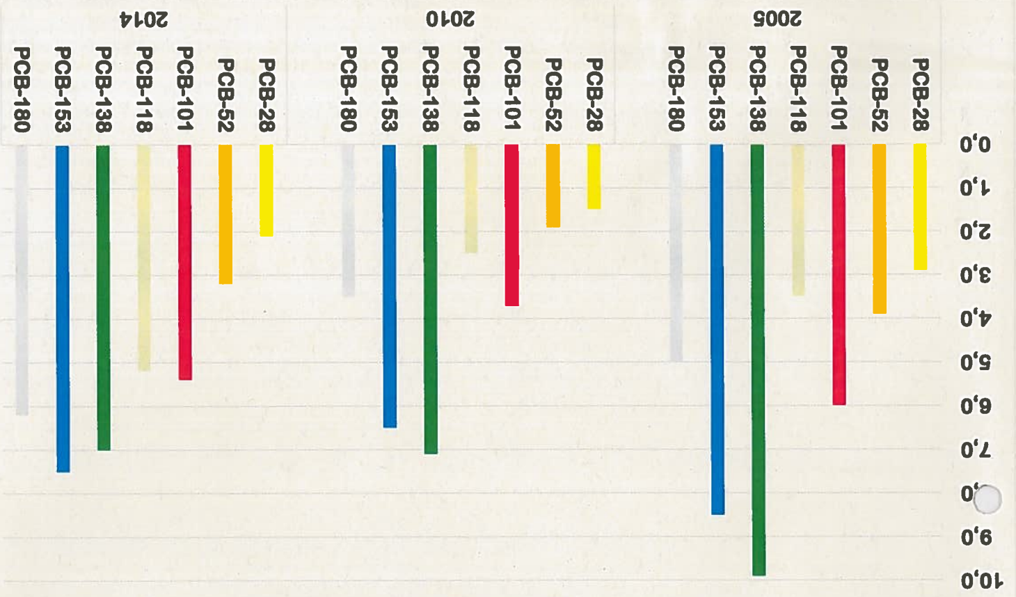
PCB-Messungen aus Proben der Schwebstoffphase [in ug/kg] des Rheins an der Meßstelle WkSt Rhein-Nord Kieve-Bimmen
