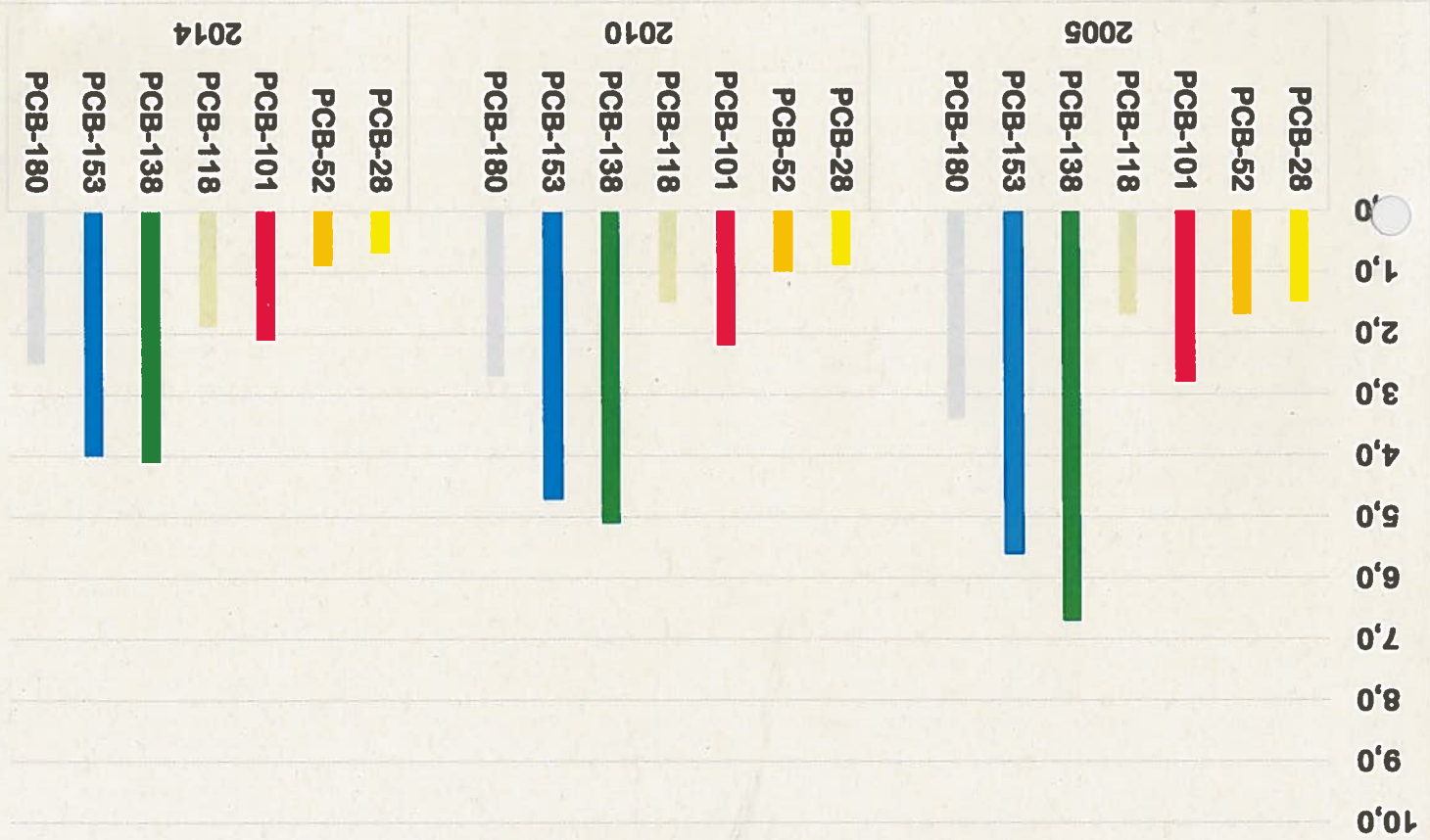
PCB-Messungen aus Proben der Schwebstoffphase [in ug/kg] des Rheins an der Meßstelle WkSt Süd/Bad Honner
